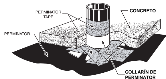
Figura 2: INSTALACIÓN DEL COLLARÍN
